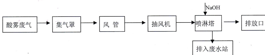
图 1--5 酸雾废气处理工艺流程图
